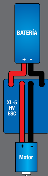
Diagrama de cableado del XL-5 HV
